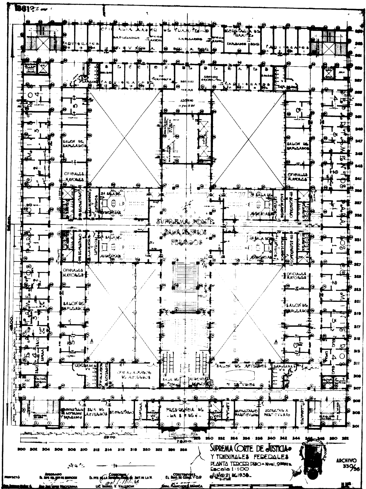
88 Plano original, en planta del tercer piso del edificio de la Av. Pino Suárez N° 2.
