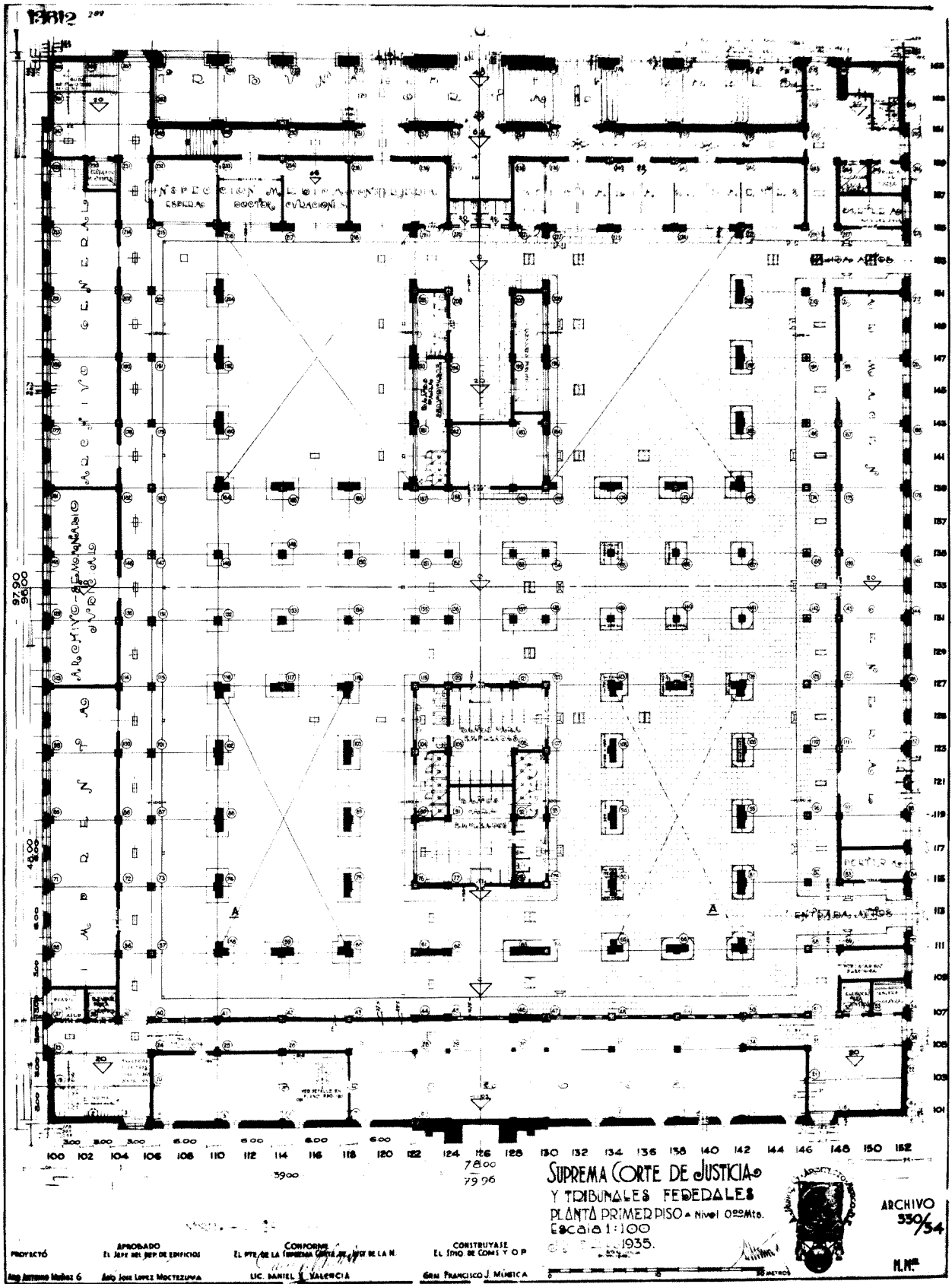
86 Plano original de la planta del primer piso, a nivel de banqueta, Av. Pino Suárez N° 2.
