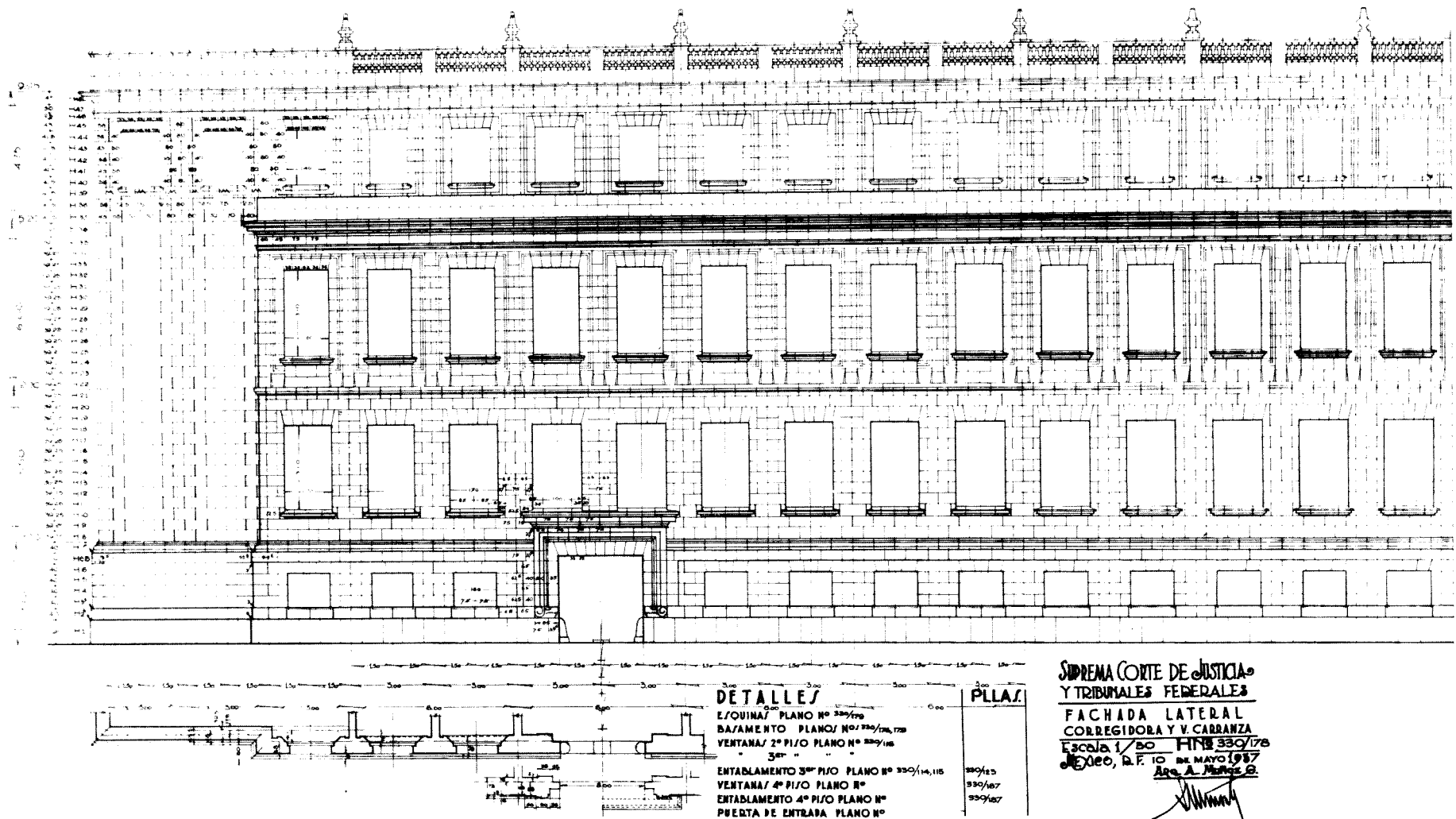
91 Plano original del alzado de la fachada sur del edificio de Pino Suárez N° 2.
